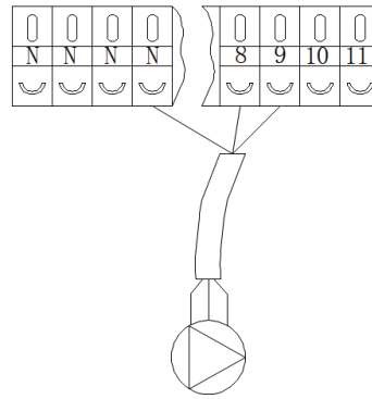
2# elektromagnetisches Drei-Wege-Ventil
