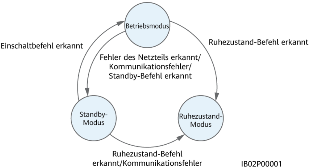
Abbildung 2-17 Umschaltung des Arbeitsmodus
