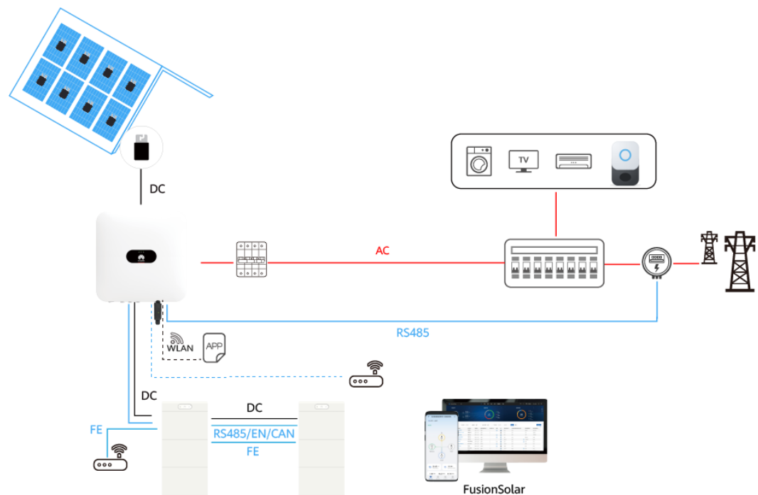
Abbildung 2-7 Netzgekoppeltes Szenario
