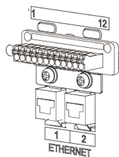
Abbildung 5-5 Signalanschluss
