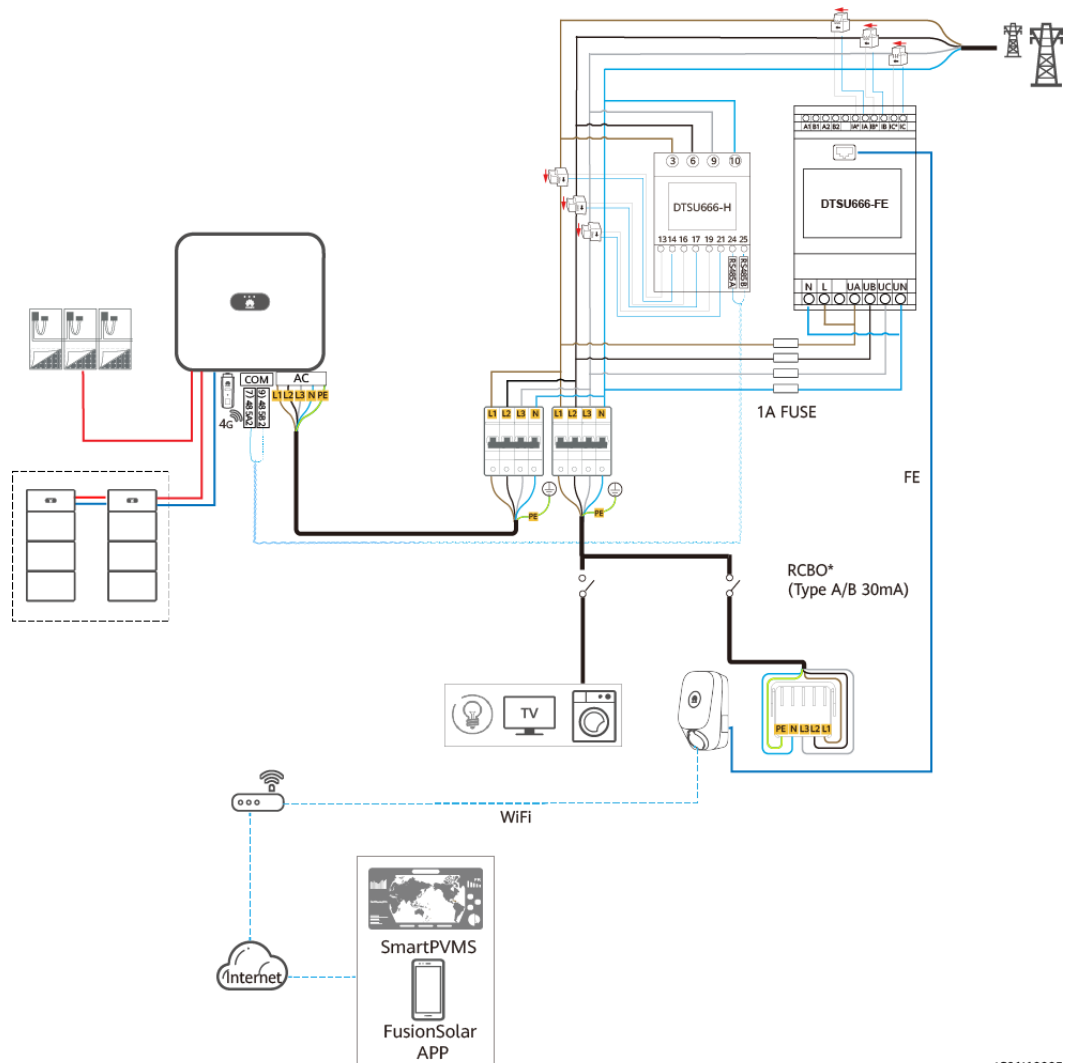
Abbildung 3-6 PV+Wallbox/PV+ESS+Wallbox (RS485-Stromzähler & FE Meter & Nicht-WLAN/FE Smart Dongle)
