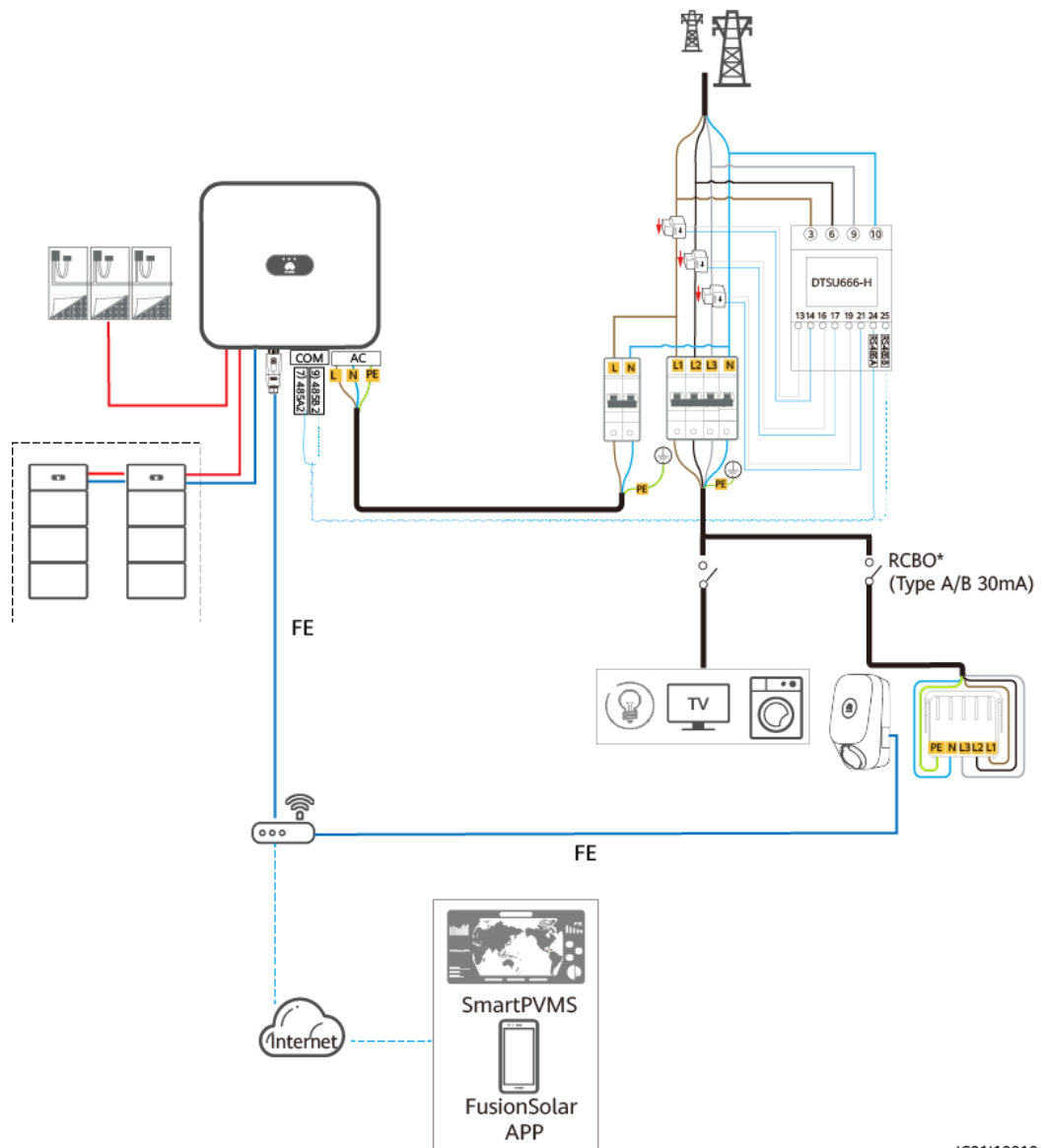
Abbildung 3-5 PV+Wallbox/PV+ESS+Wallbox (RS485-Zähler & WLAN/FE Smart Dongle, einphasiger Wechselrichter mit dreiphasiger Wallbox)
