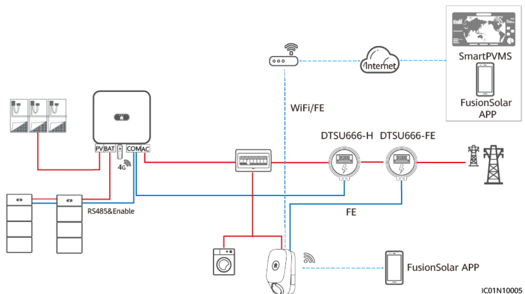
Abbildung 2-6 PV+Wallbox/PV+ESS+Wallbox (RS485-Stromzähler & FE-Stromzähler & Nicht-WLAN/FE Smart Dongle, unter Verwendung einer direkt an einen FE-Stromzähler angeschlossenen Wallbox als Beispiel)
