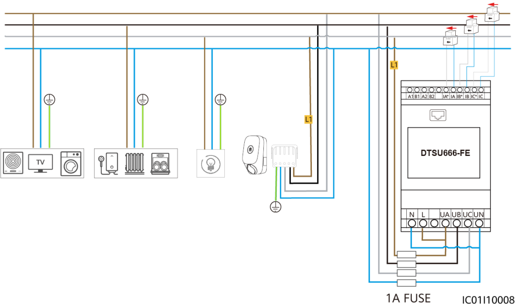
Abbildung 3-7 Anschluss der L1-Wallbox an den Phasenleiter mit der Mindestlast
