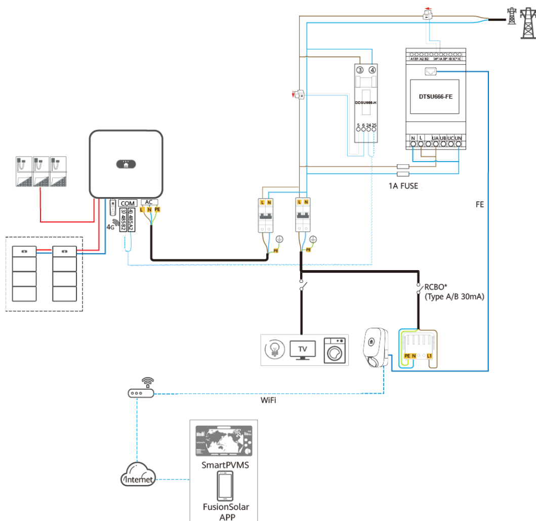
Abbildung 3-8 Schaltplan für einphasiges System (TN & TT einphasig)
