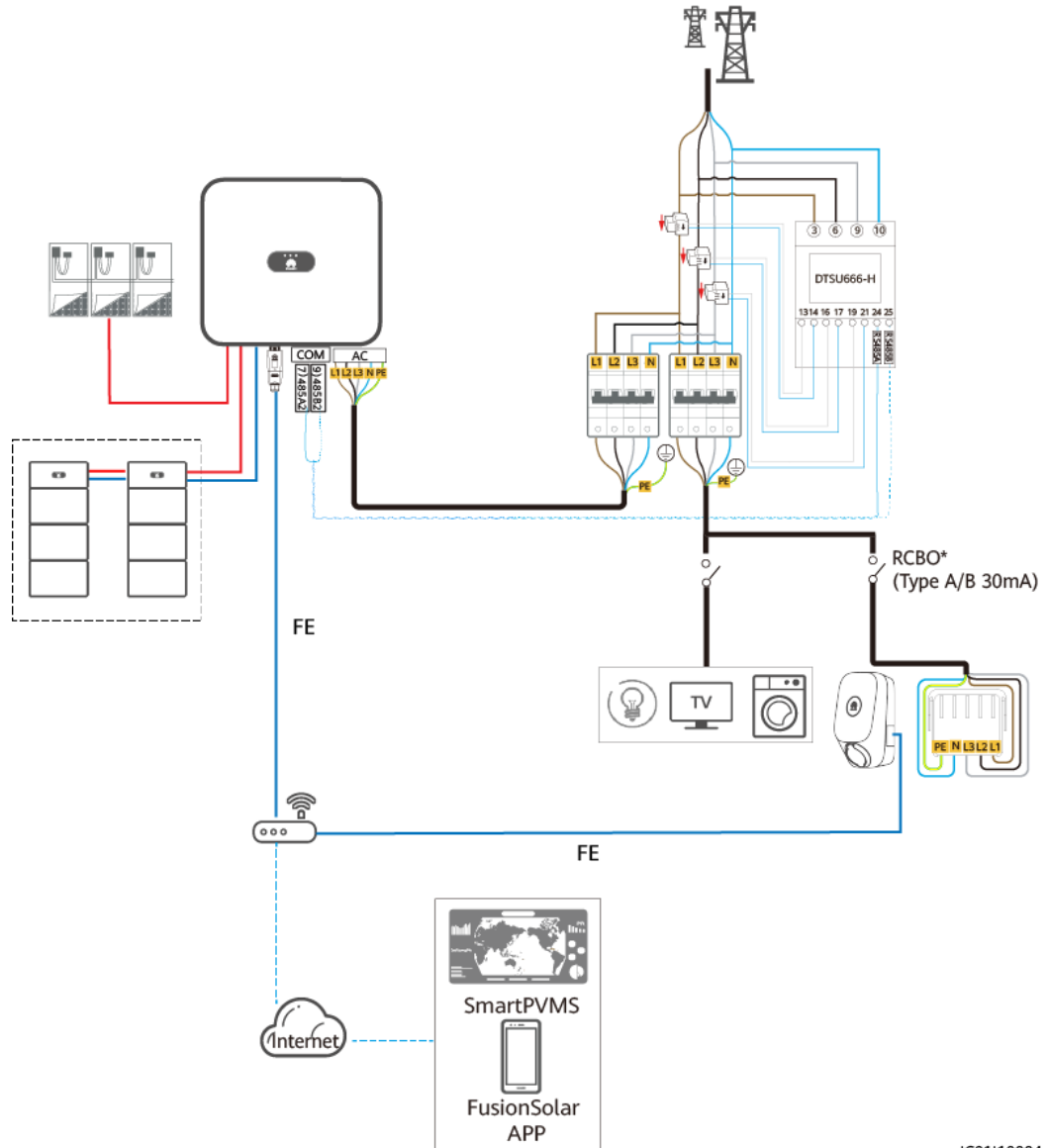
Abbildung 3-4 PV+Wallbox/PV+ESS+Wallbox (RS485-Zähler & WLAN/FE Smart Dongle, dreiphasiger Wechselrichter mit dreiphasiger Wallbox)
