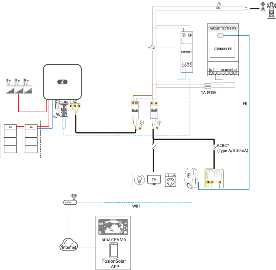
Abbildung 3-9 Schaltplan für einphasiges System (230 V L-L)
