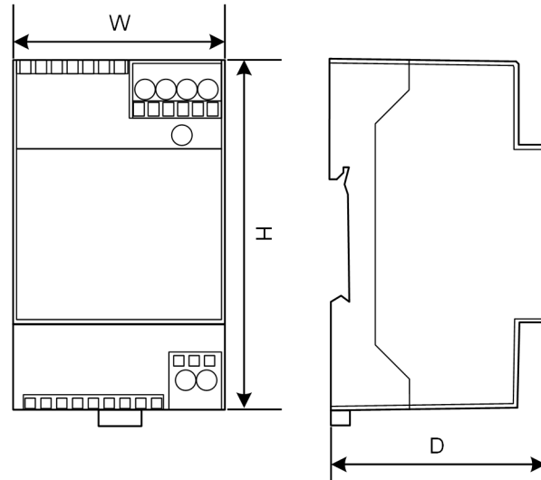
Abb. 5-6: Schematische Darstellung, Abmessungen in Millimeter
