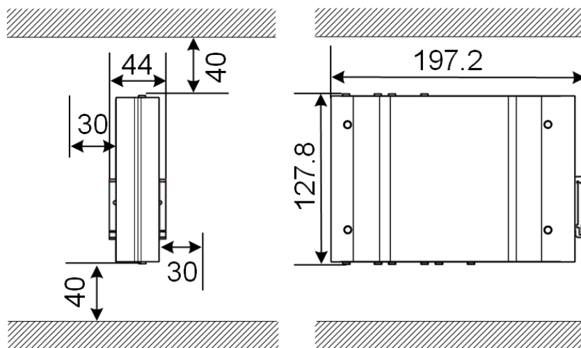
Kuva 3-3: Tilan tarve (mitat millimetreinä) asennettaessa kytentäkaappiin
