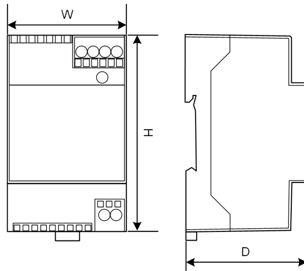
Fig. 5-6: Representação esquemática, dimensões em milímetros
