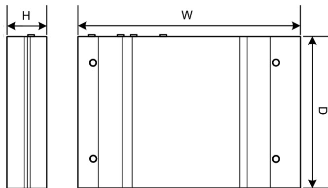
Fig. 5-5: Représentation schématique, dimensions en millimètres
