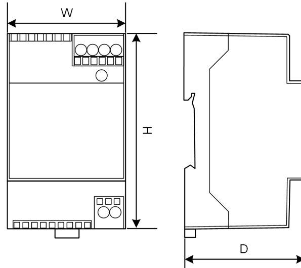
Εικ. 5-6: Σχηματική αναπαράσταση, διαστάσεις σε χιλιοστά
