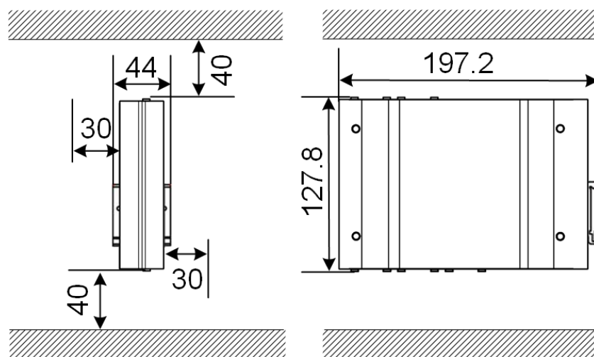
Fig. 3-3: Plassbehov (mål i mm) ved koblingsskapmontering
