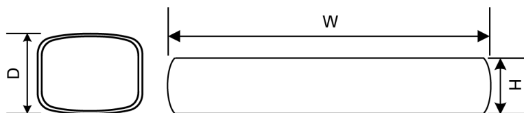
Εικ. 5-4: Σχηματική αναπαράσταση, διαστάσεις σε χιλιοστά
